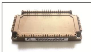
A-FLY ID:AF-M262 MODEL:7MBR75VR120-50
